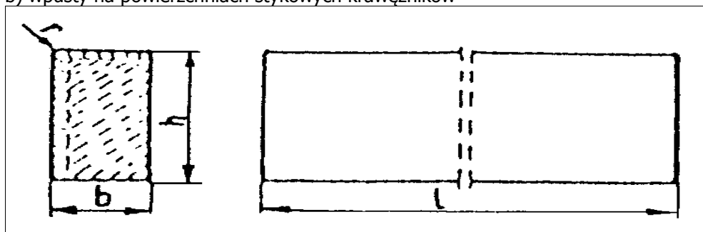
Rys. 1. Wymiarowanie krawężników
