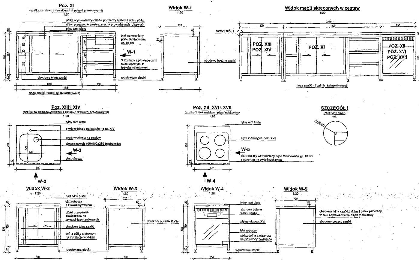
ZAŁĄCZNIK NR 7 DO SIWZ - Rysunek złożeniowy
